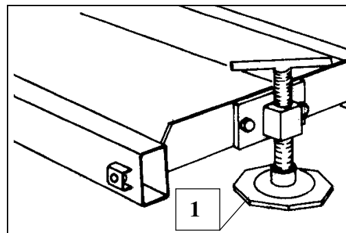
Afb. 15 Instelspil
