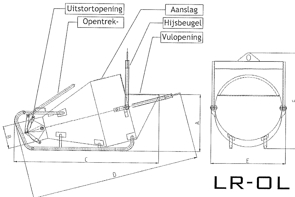
Figuur 2: Tekening betonstortkubel liggend rond model met
