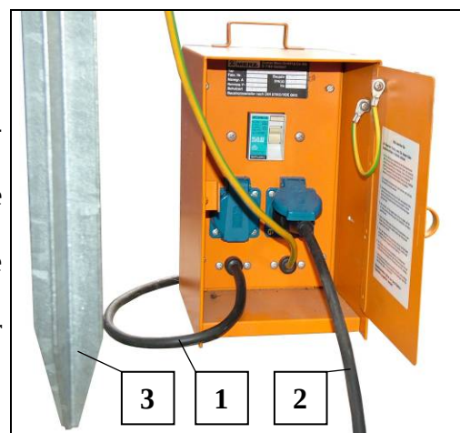
Fig. 17 Mini-bouwstroomverdeler
