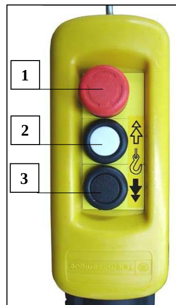
Fig. 72 Handbesturingen tweetraps
