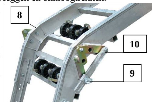
Fig. 22 Knikstuk instellen
