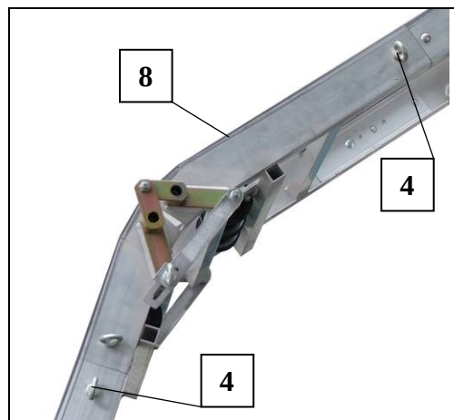
Fig. 21 Knikstuk monteren
