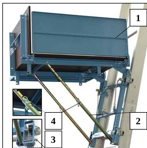
Fig. 47 Vario-platform
