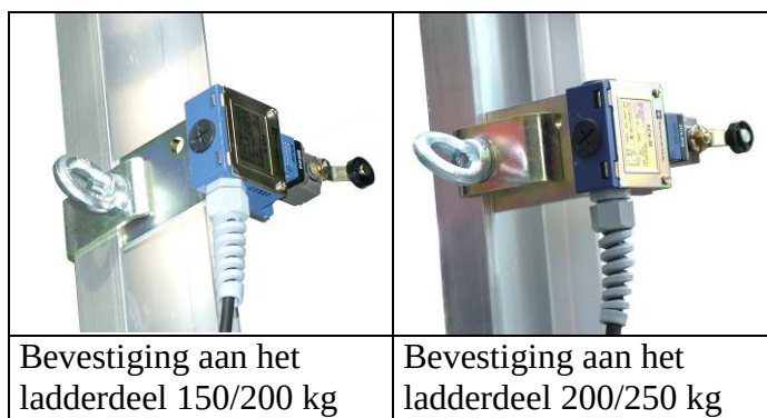
Fig. 33 Bovenste eindeloopschakelaar aanbrengen
