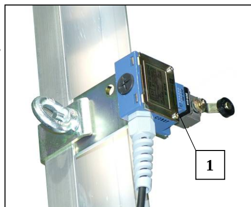
Fig. 10 Eindeloopschakelaar boven
