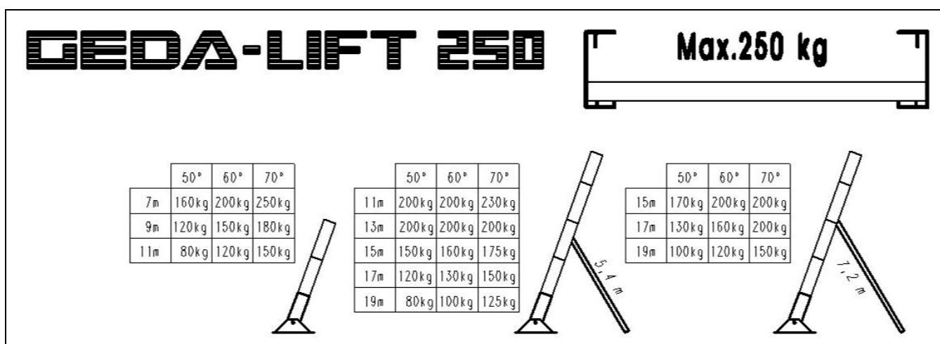
Fig. 25 Belastingstabel voor ladderdelen 200/250 kg
