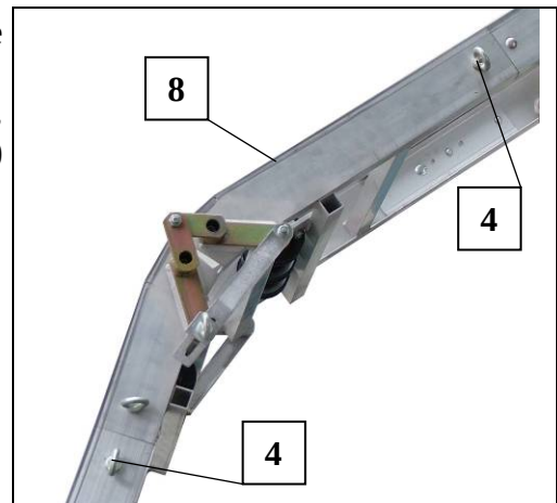
Fig. 21 Knikstuk monteren
