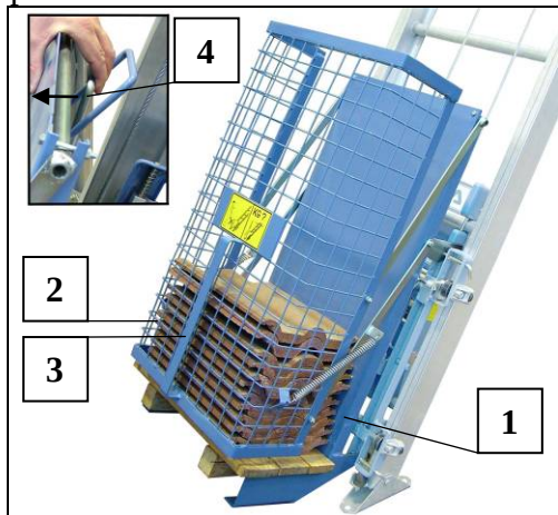
Fig. 56 Pannenplateau
