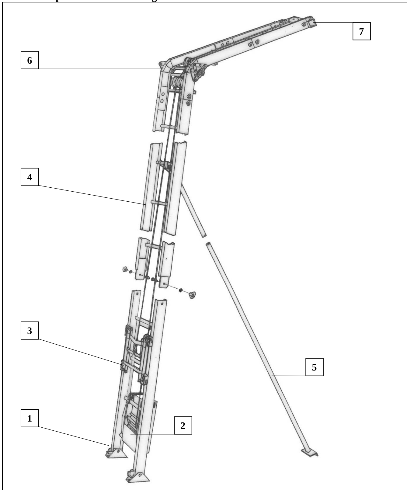
Fig. 4 GEDA-LIFT
