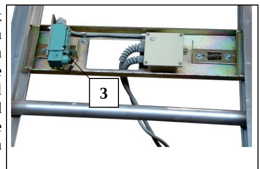
Fig. 70 Flexibele schakelaar
