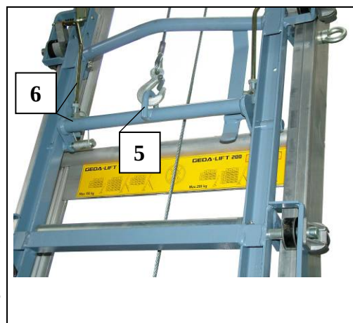
Fig. 38 Kabel aan slede vasthaken
