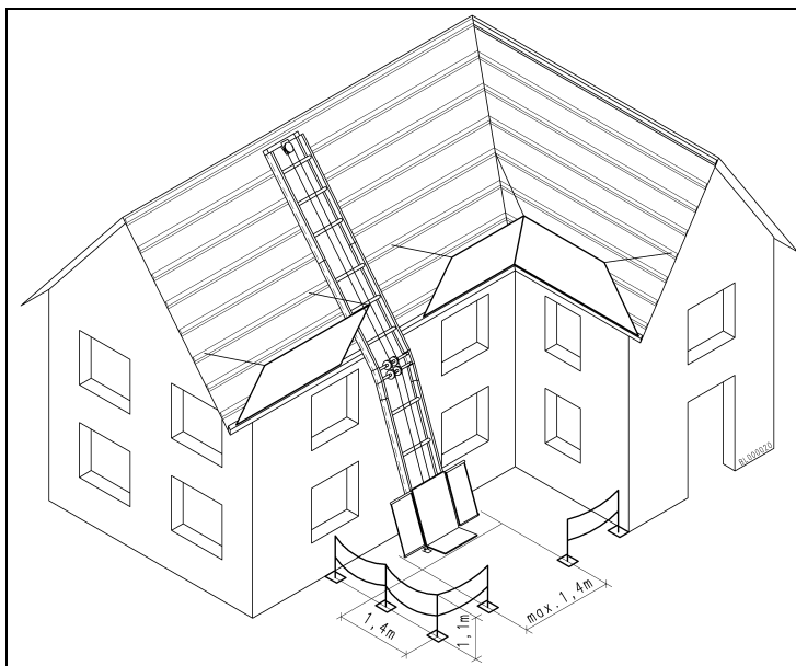
Fig. 3 Afzetten van de gevarenzone
