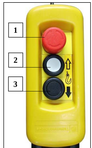
Fig. 71 Handbesturing ééntraps
