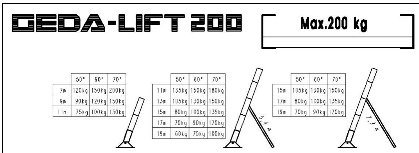
Fig. 24 Belastingstabel voor ladderdelen 150/200 kg
