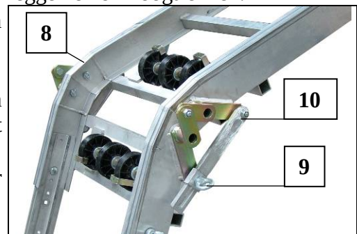
Fig. 22 Knikstuk instellen
